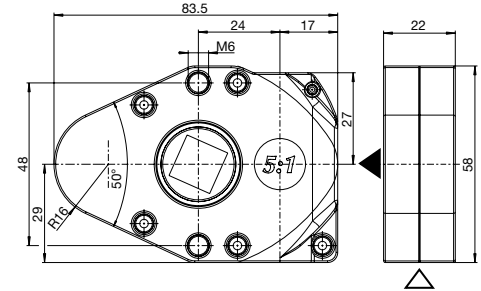
Gehäuseform A (TK 48 mm)
